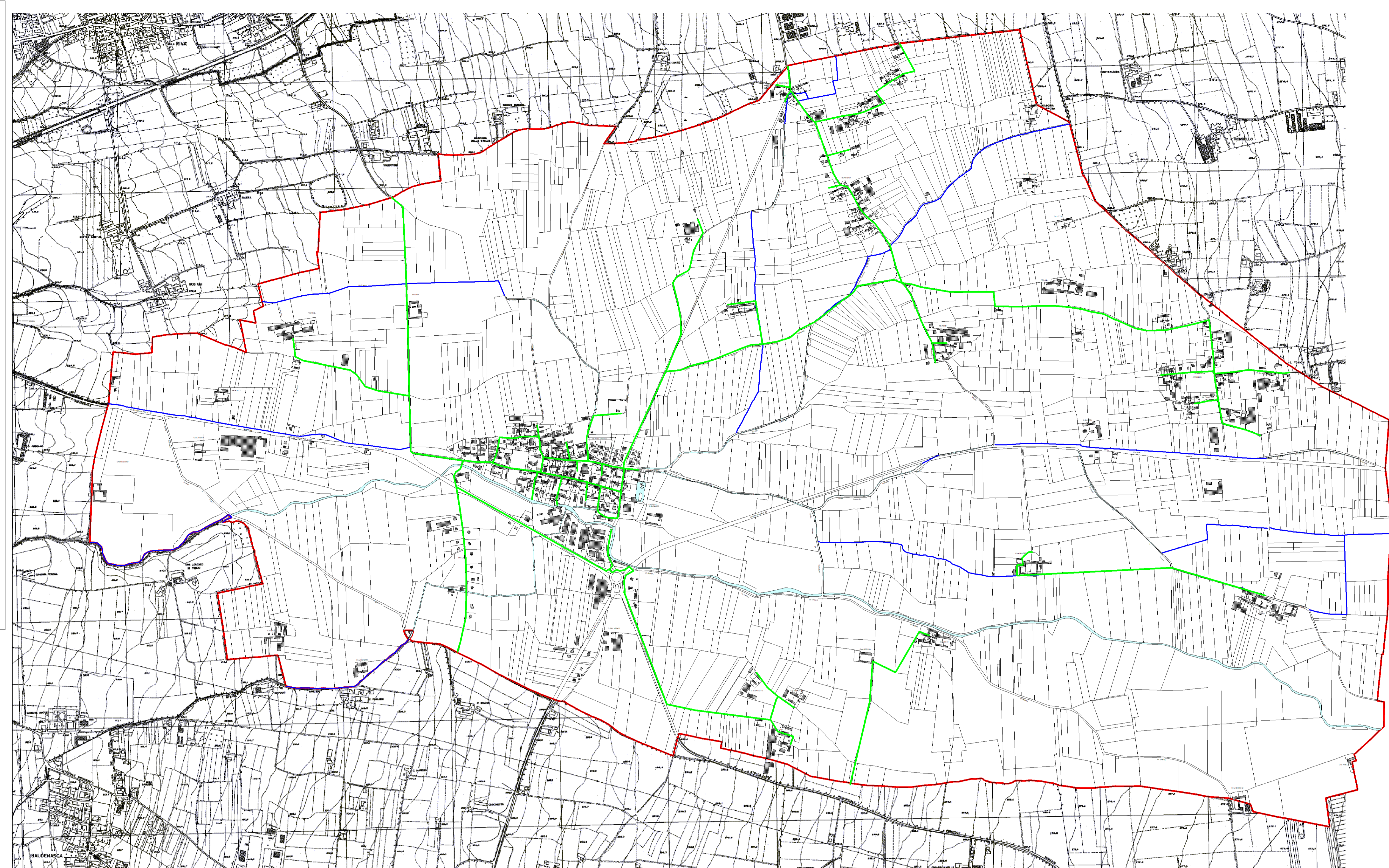
INFRASTRUTTURE A RETE "ACQUEDOTTO" - STATO DI FATTO (SCALA 1:10.000)
